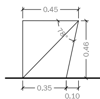
Perfil
