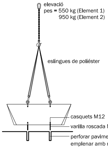
Alçat frontal
