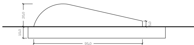
Alçat lateral
