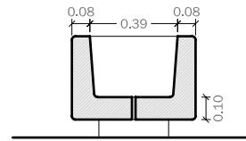
Sección
