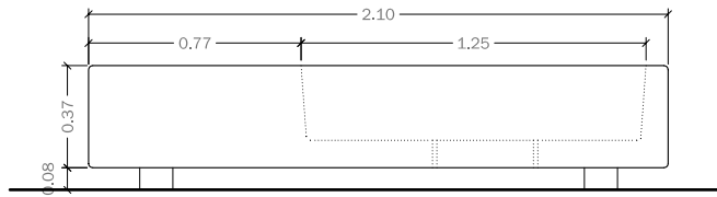
Alzado
