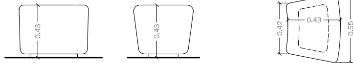
Alzado
