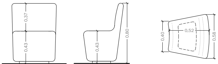
Alzado
