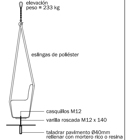
Alzado lateral
