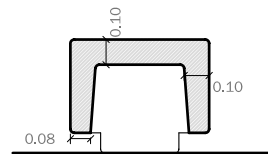
Sección
