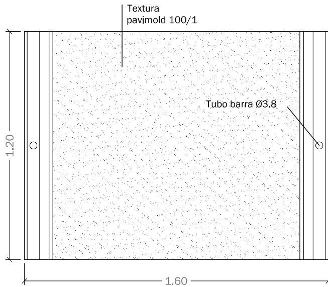
Planta
