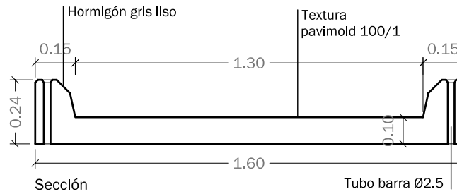
Sección
