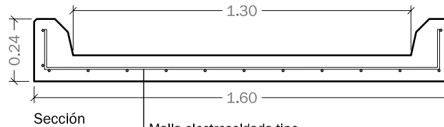
Sección
