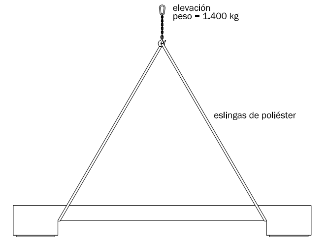
Sistema de Fijación Apoyado
