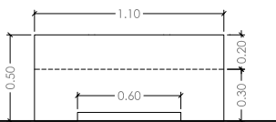
Alzado posterior
