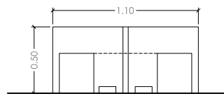
Alzado frontal
