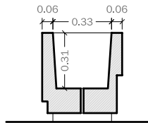
Secció
