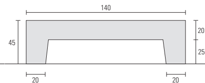
SECCIÓN
