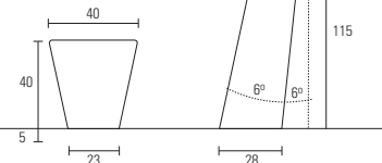
PERFIL (banco-respaldo)
