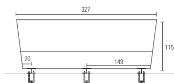
FRONTAL (banco-respaldo)
